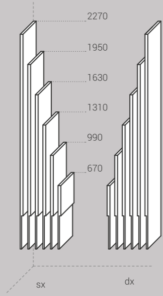
spalle con scanco per basi sospese h. 320, h. 480 side panels with undercut for suspended bases h. 320, h. 480
