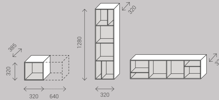
→ PENSILI A GIORNO / OPEN WALL UNITS
